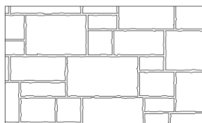
PERM_LAFITT50 Appareil irrégulier avec 50% grosses pierres
