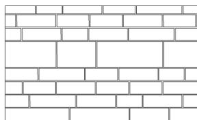
PERM_P_CINCO_C2 Appareil irrégulier avec brique Cinco
