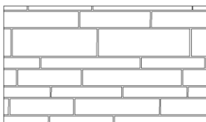
PERM_LEXA_B Appareil irrégulier avec 33% grosses pierres
