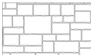
PERM_LAFITT10 Appareil irrégulier avec 10% grosses pierres
