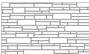
PERM_LAMINA_AB-1 Appareil en panneresse avec 20% grosses pierres
