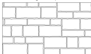
PERM_LAFITT_E2 Appareil irrégulier avec petites et moyennes pierres
