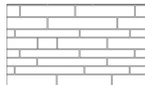
PERM_LEXA_D Appareil irrégulier avec petites et moyennes pierres
