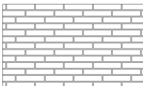
PERM_MELVILLE_NORMAN_B2 Appareil en panneresse modifié
